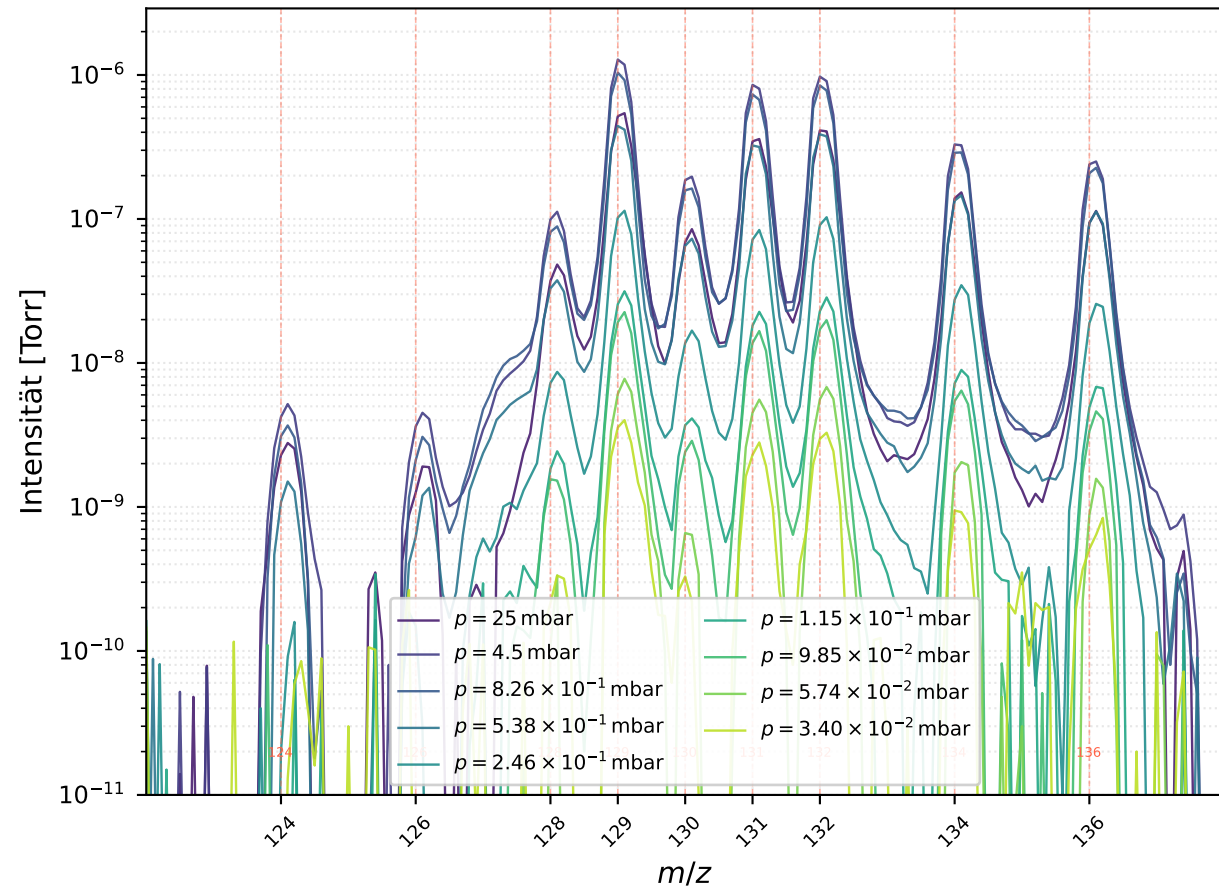
(a) \text{Xe}^+ — einfach ionisiert ( m/z = A )
