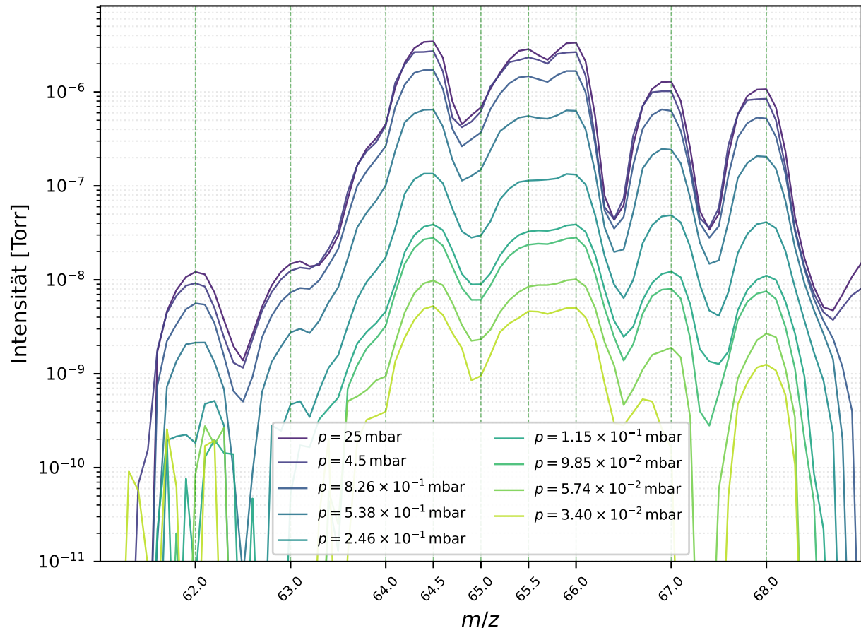
(b) \text{Xe}^{2+} — doppelt ionisiert ( m/z = A/2 )
